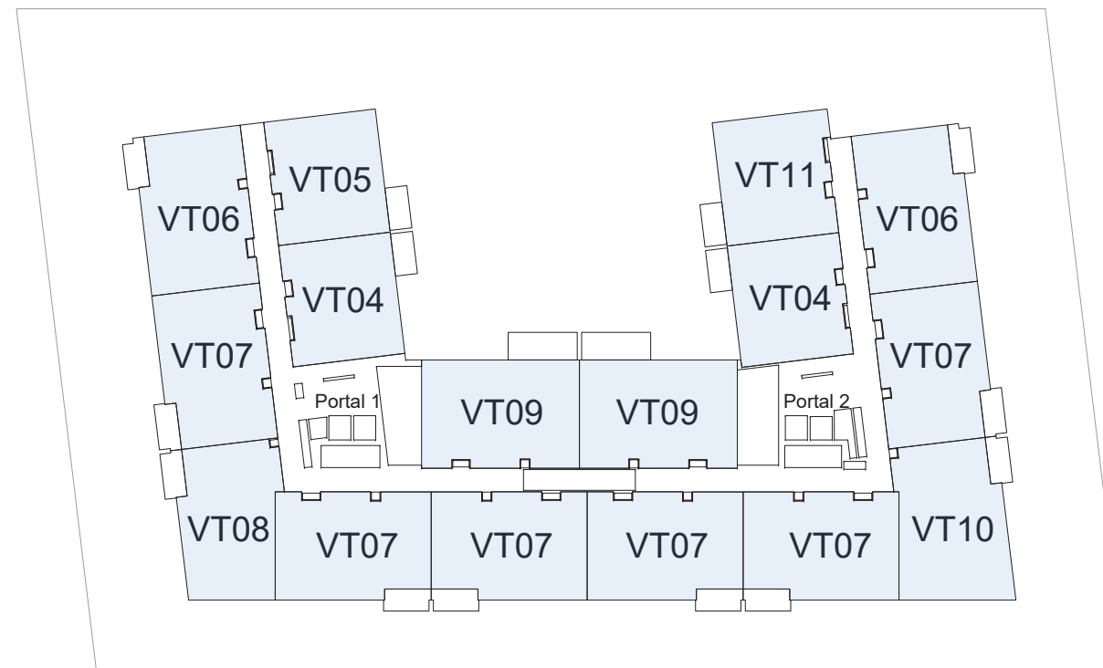
PLANTA TIPO (1ª A 3ª)
