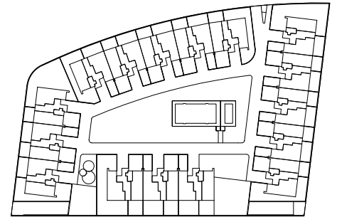
PLANTA BAJA
